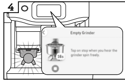
4 Mahlwerk leer laufen lassen
